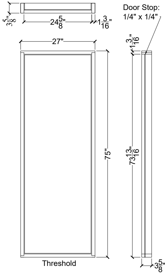
Door Jamb
