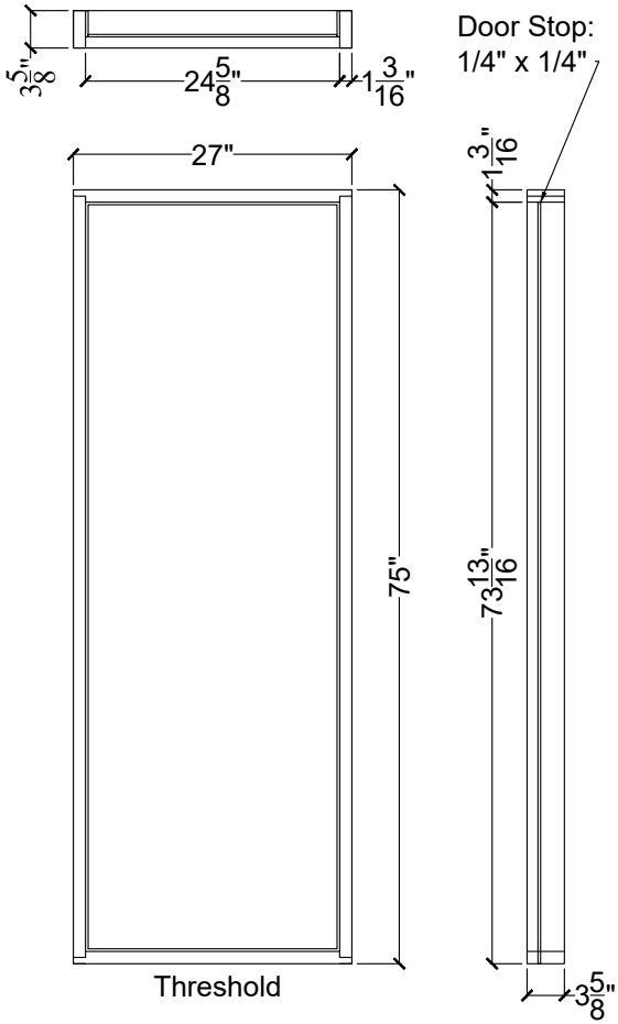
Door Jamb
