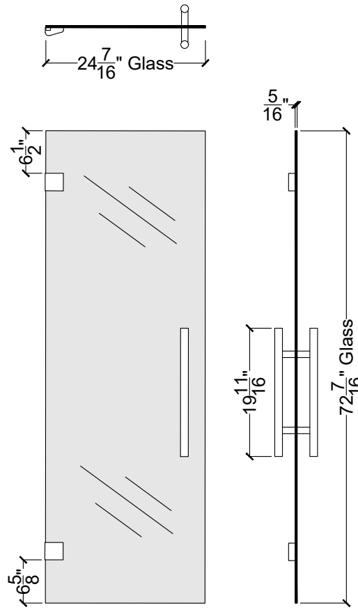
Door
