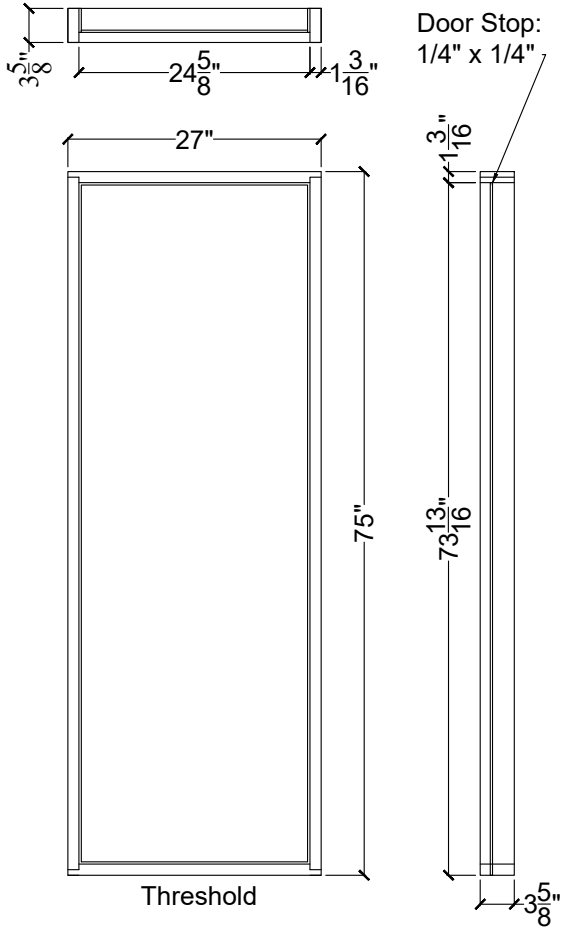
Door Jamb
