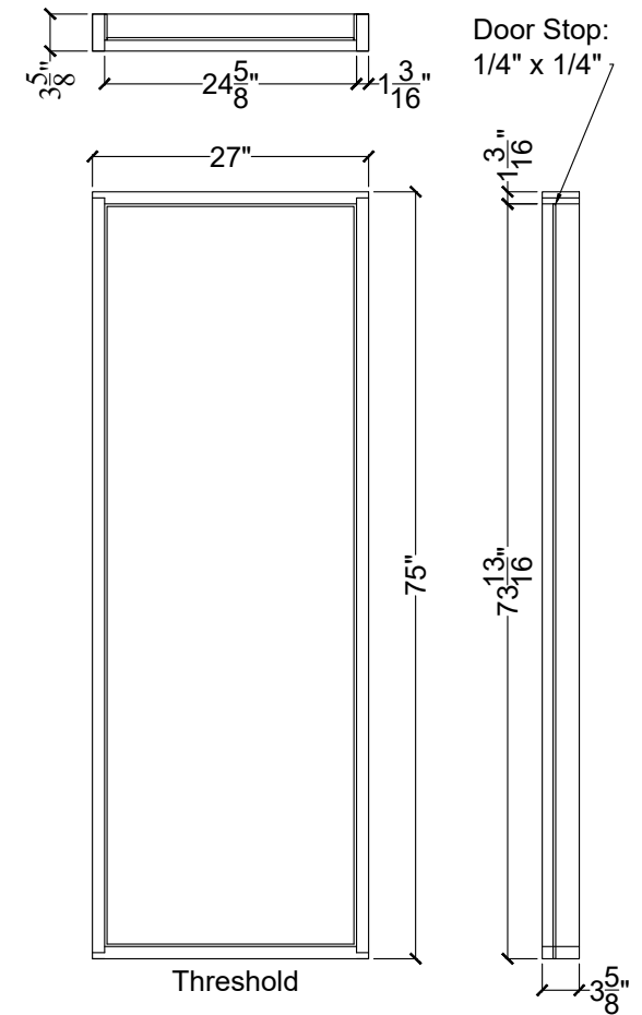
Door Jamb
