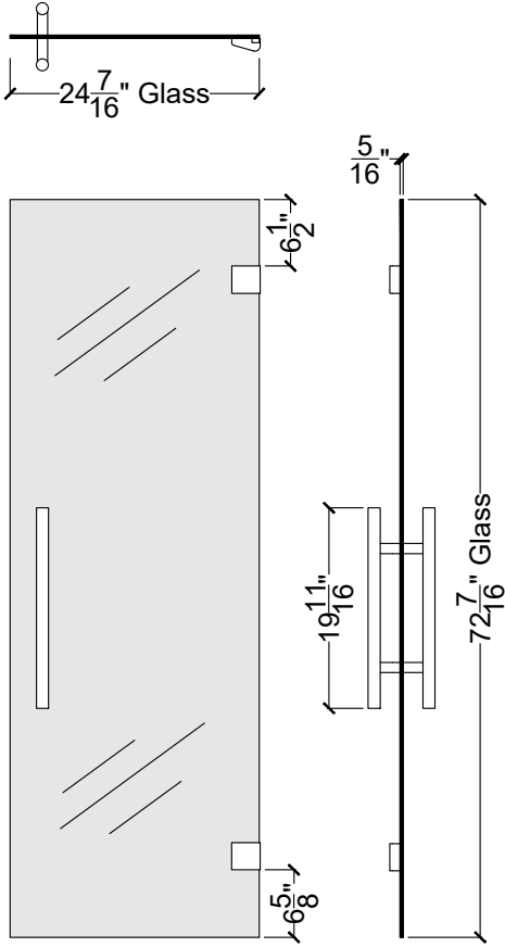
Door
