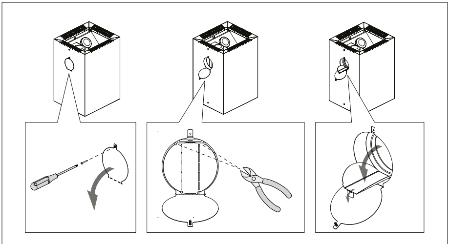
6. Die hintere Anschlussöffnung
