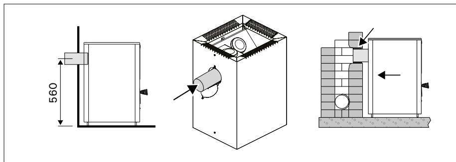
9. Anschluss des Ofens an einen gemauerten Rauchfang über die hintere Anschlussöffnung
