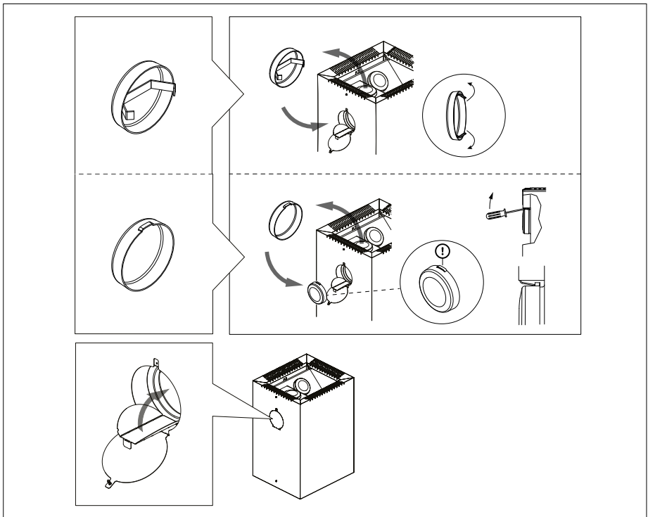
7. Die obere Anschlussöffnung
