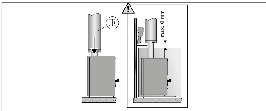
11. Anschluss des Ofens an einen Harvia-Edelstahlschornstein
