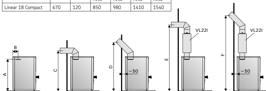
8. Position der oberen und hinteren Anschlussöffnungen
