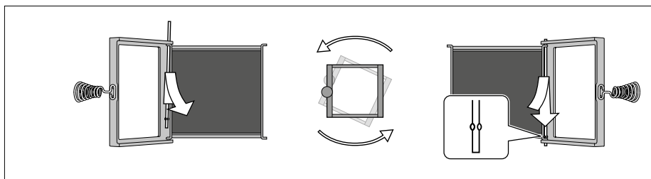
12. Änderung der Öffnungsrichtung der Ofentür
