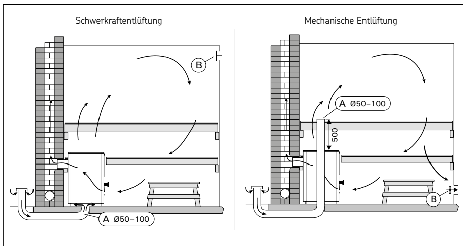
3. Belüftung der Saunakabine
