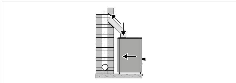
10. Anschluss des Ofens an einen gemauerten Rauchfang über die obere Anschlussöffnung
